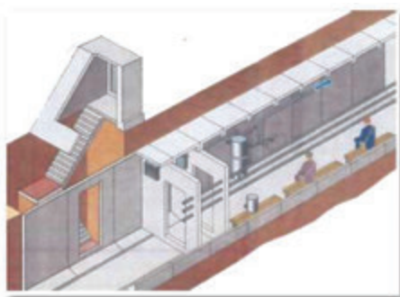
ПРИСПОСОБЛЕНИЕ ОБЩЕГО КОЛЛЕКТОРА ПОД УКРЫТИЕ
